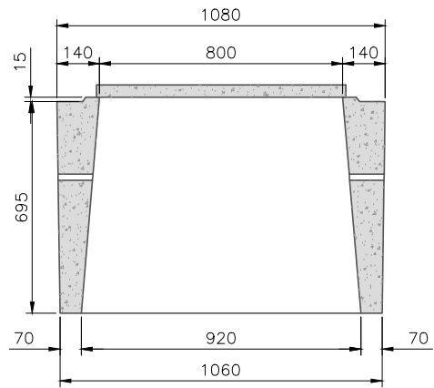
Módulo normal
